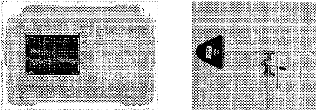
Fig. 10. Analizador de espectro y antena
