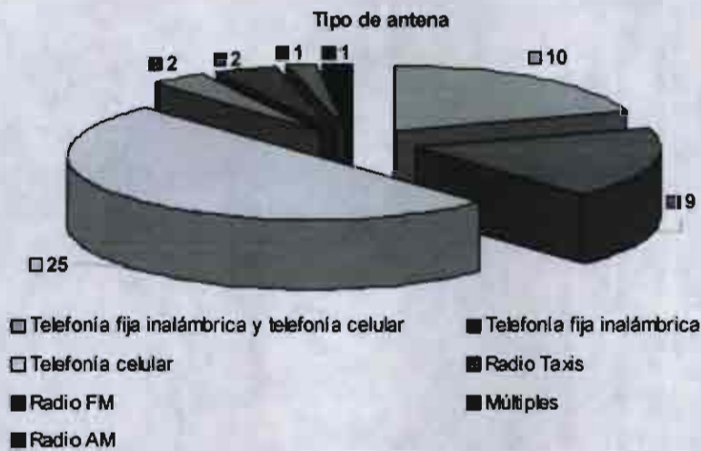
Fig. 24. Tipos de antenas medidas
