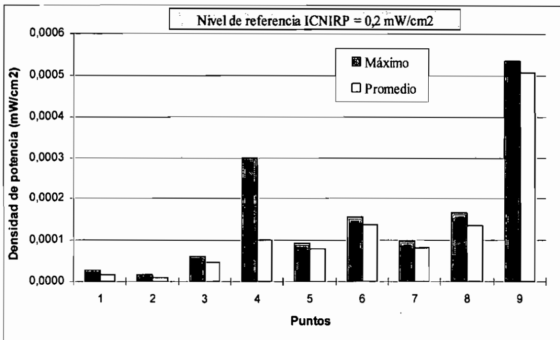
Fig. 17. Valores máximos y promedios obtenidos para todos los puntos
