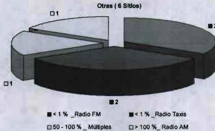
Fig. 30. Valores máximos en otros sitios con respecto a 0.2 mW/cm 2
