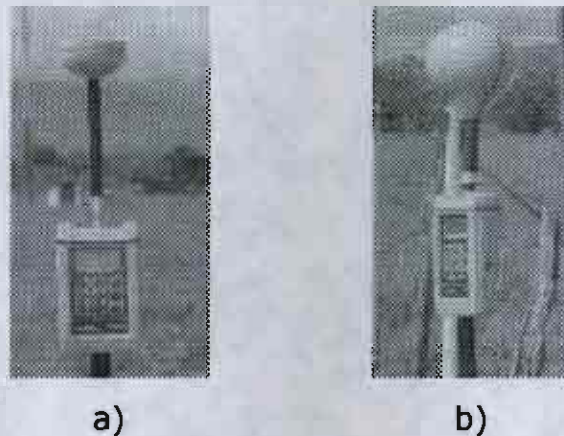
Fig. 12. Sensores de campo a) eléctrico y b) magnético
