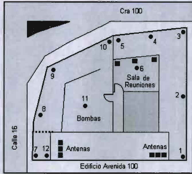
Fig. 31. Vista de planta del sitio de medición
