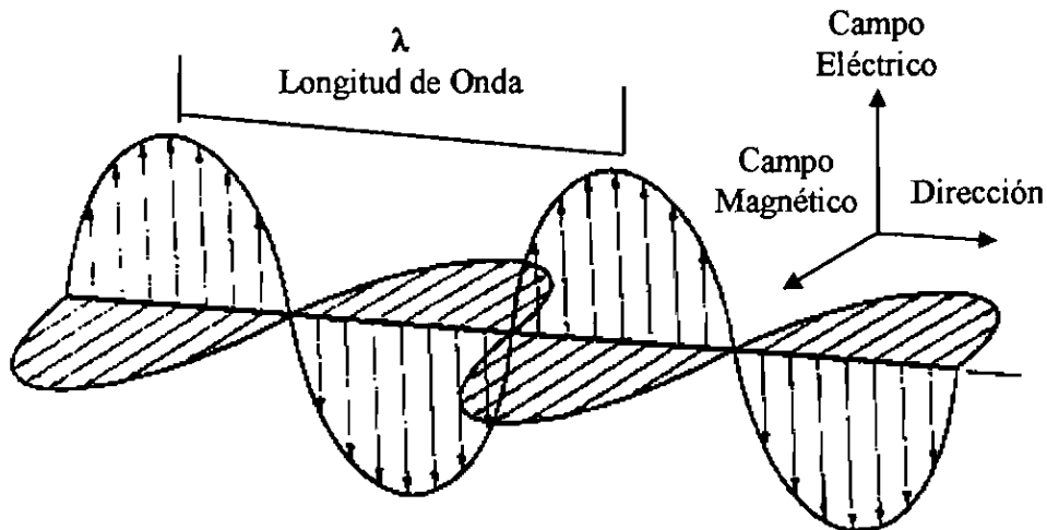
Fig. 4. Propagación de una onda electromagnética
