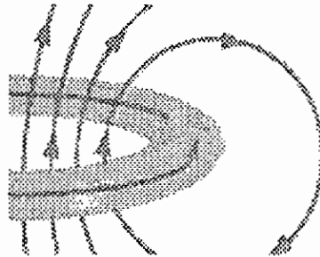
Fig. 3. Líneas de campo magnético
