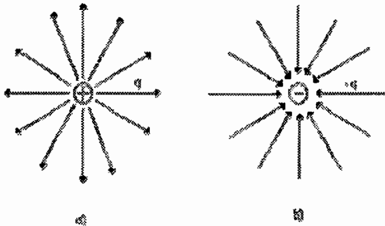
Fig. 2. Líneas de campo eléctrico de una carga puntual a) positiva y b) negativa
