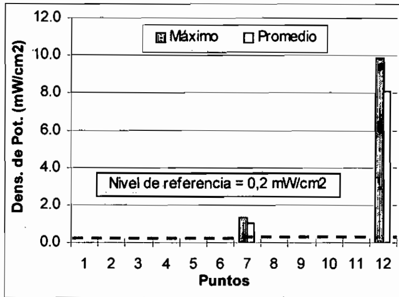
Fig. 33. Valores máximos y promedios de densidad de potencia
