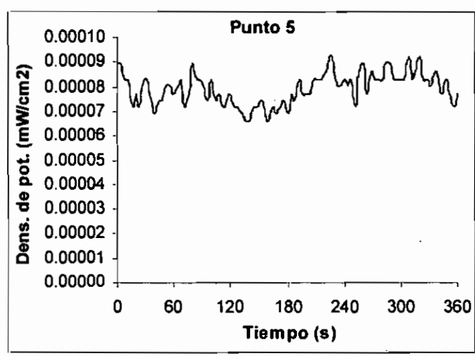
Fig. 16. Densidad de potencia en función del tiempo para un punto
