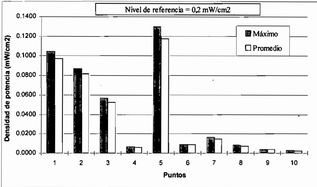
Fig. 37. Valores máximos y promedios de densidad de potencia
