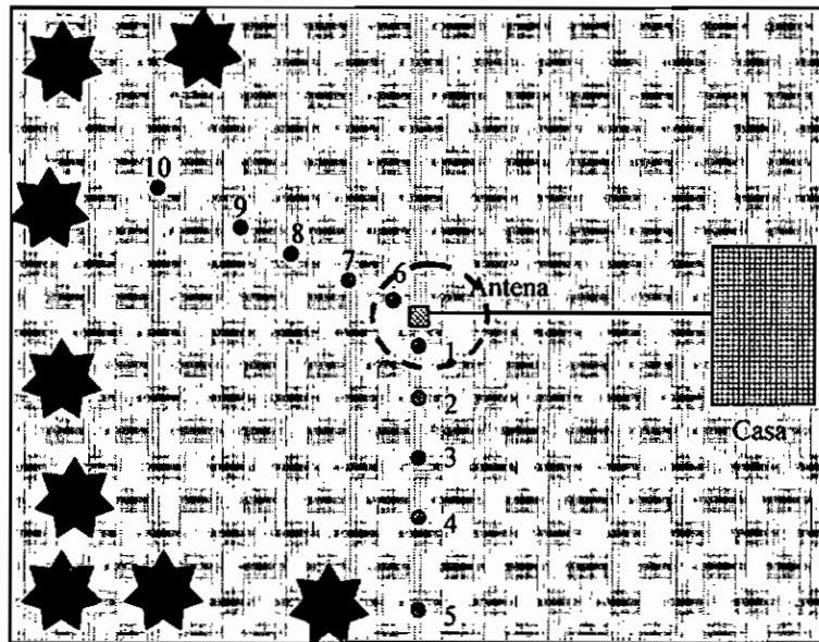
Fig. 34. Vista de planta del sitio de medición
