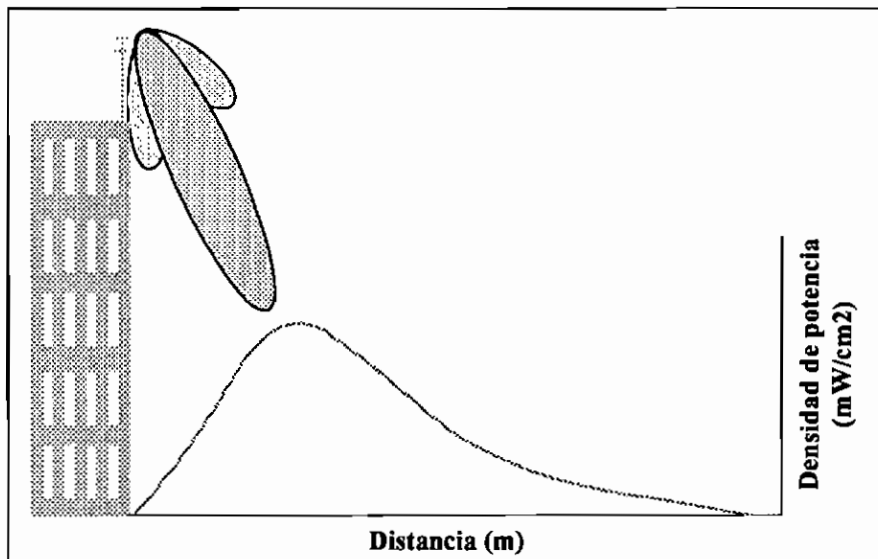
Fig. 9. Radiación de una antena de telefonía celular
