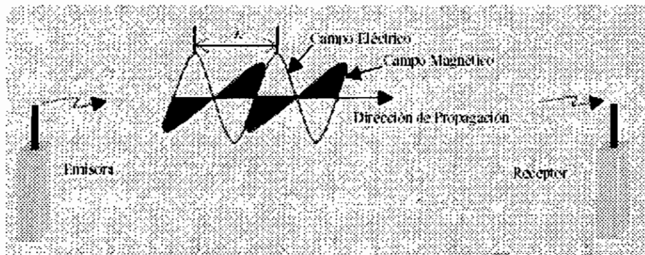
Fig. 1. Propagación de una onda electromagnética
