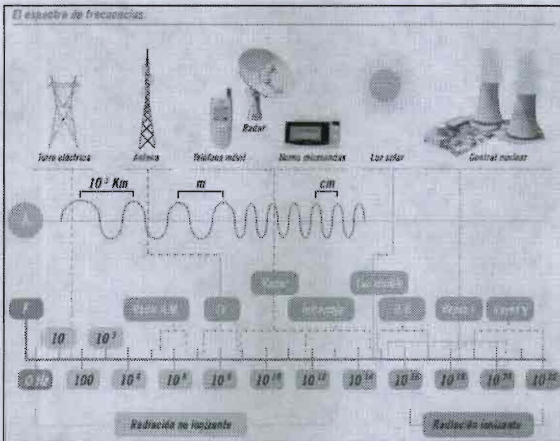
Fig. 5. Espectro electromagnético
