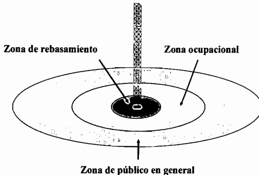
Fig. 22. Zonas de exposición a campos electromagnéticos
