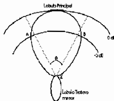
Fig. 7. Ancho de haz de la antena
