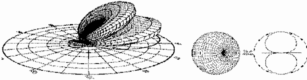
Fig. 6. Diagrama de radiación de una antena
